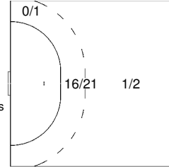
9 VORI Igor
