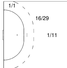
22 LIJEWSKI Marcin
