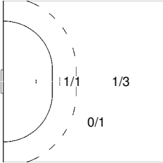
2 JASZKA Bartlomiej
