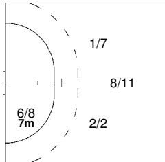
11 STEFÁNSSON Ólafur
