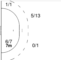
5 VÍTEK Jirí
