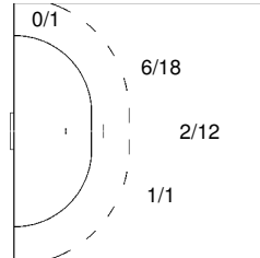
7 MARKOVIC Zarko
