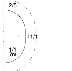
8 PETERSSON Johan
