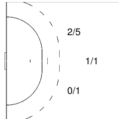
20 REZNÍČEK Tomás
