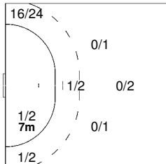
24 LINDBERG Hans
