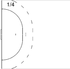
3 VASILIEU Aliaksei
