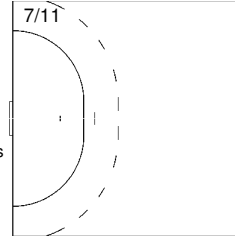
4 KUCHCZYNSKI Patryk
