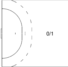
6 BACKOVIC Ognjen
