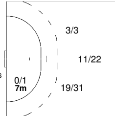
8 BIELECKI Karol
