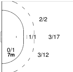
15 HARBOK Siarhei
