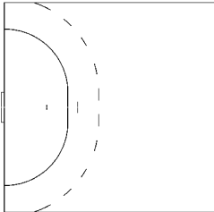
19 POGORELOV Serguei
