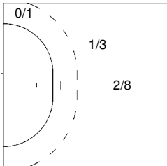
21 MIKECI Marek
