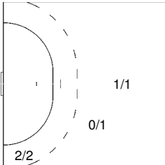
5 KLEIN Dominik
