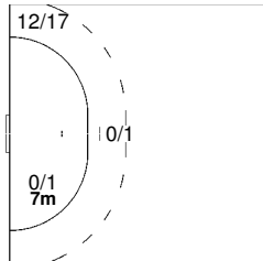
13 HORVAT Zlatko
