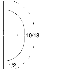
13 JURECKI Bartosz
