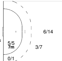
15 KJELLING Kristian
