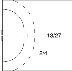
5 SULC Frantisek
