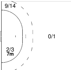
9 LENNARTSSON Jan
