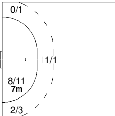
19 TLUCZYNSKI Tomasz
