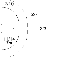
7 KAVTICNIK Vid
