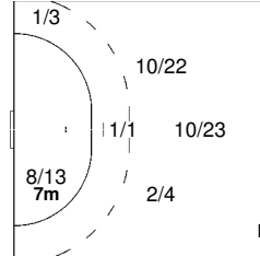
5 ANDERSSON Kim
