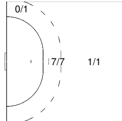
8 PREIß Sebastian
