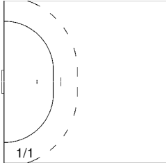
10 DIBIROV Timur
