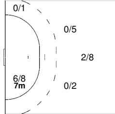
13 IGROPULO Konstantin
